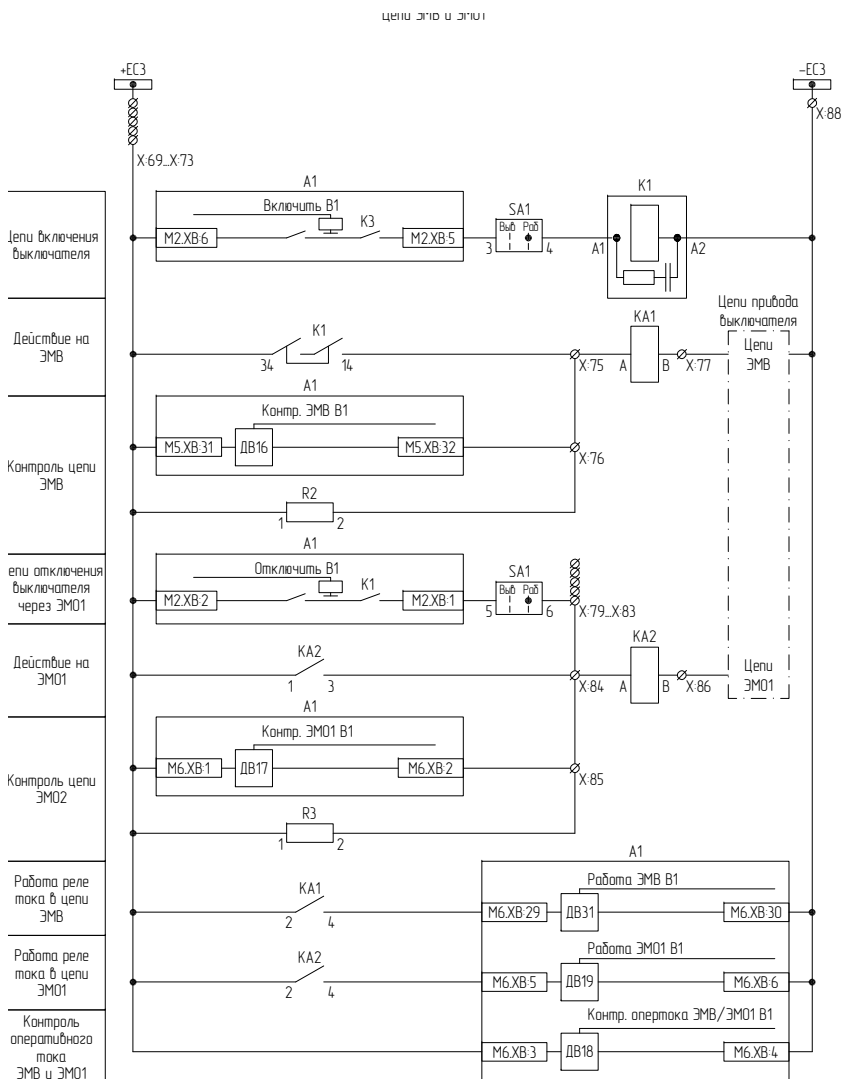
Рисунок В.3 – Схема электрическая принципиальная (часть 3)
