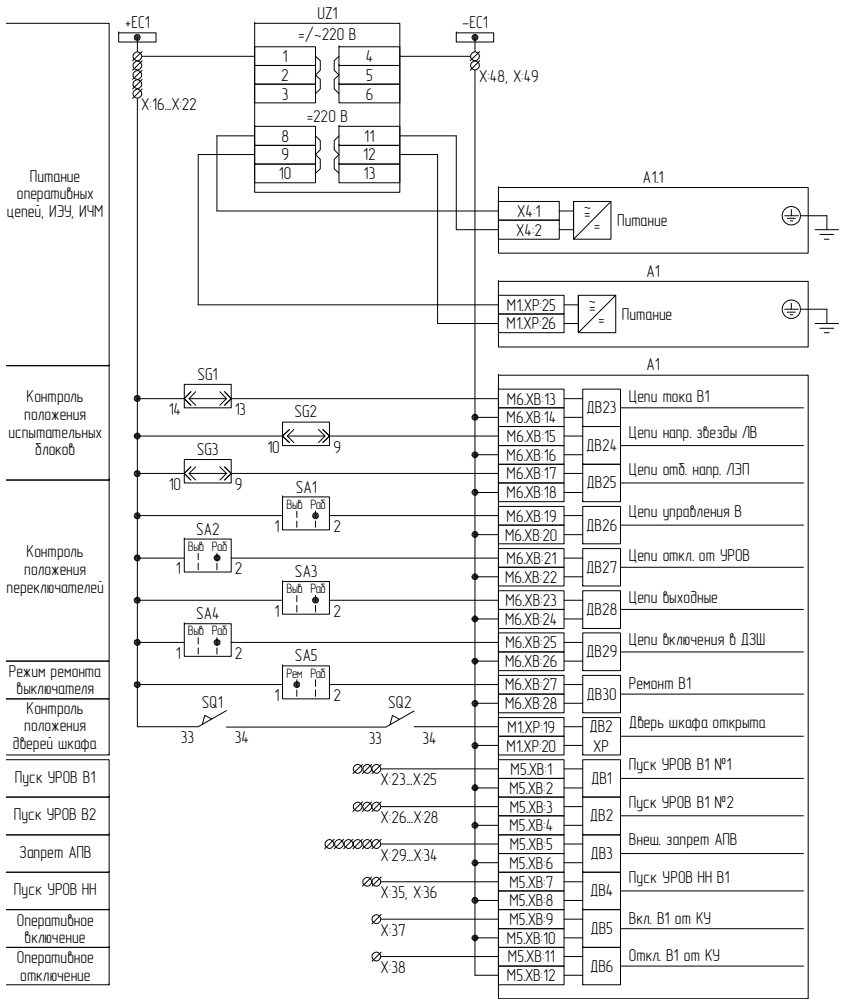
Рисунок В.2 – Схема электрическая принципиальная (часть 2)
